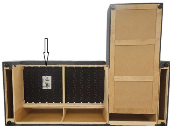
1. Sisältää: 4 osaa, 12 pulttia, 4 mutteria, 4 aluslevyä, 1 muovijalka
